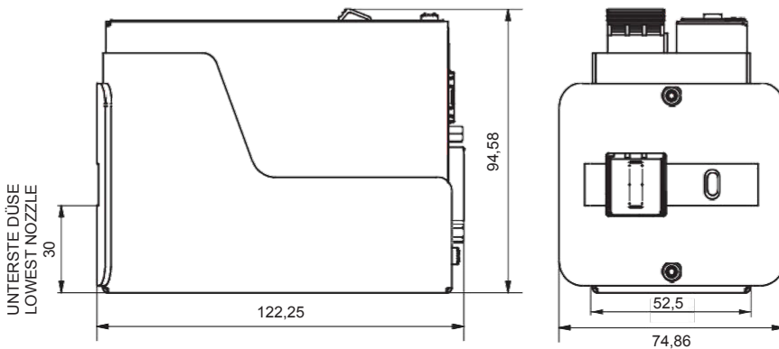
Schéma dimensionnel
